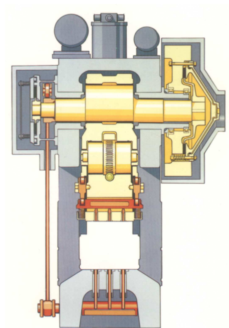
Figure 3 : Schéma de la presse mécanique à excentrique
