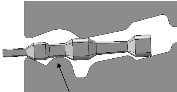
Figure 6 : Image de l'opération de cambrage
